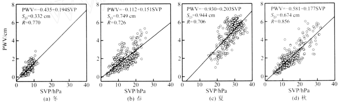
图2 各个季节PWV与SVP之间关系的散点图和对应的回归曲线
