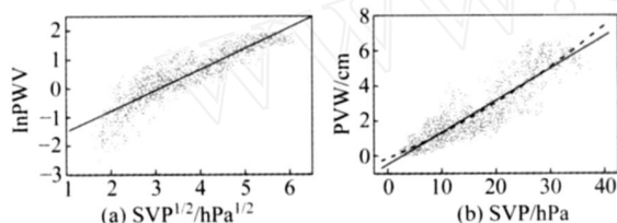
图 1 \ln PWV 与 SVP^{1/2} 之间以及 PWV 与 SVP 之间的关系
