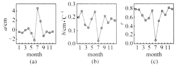
图3 月经验系数 a 、 b 以及相关系数 R 的年变化
