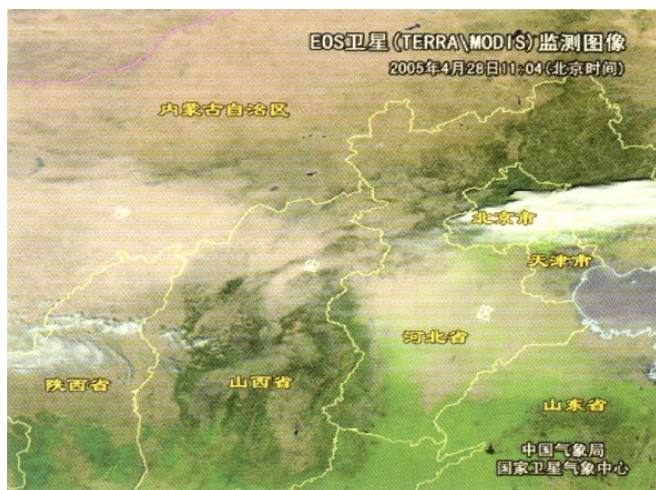
图1 2005年4月28日11时EOS卫星沙尘天气监测图像
