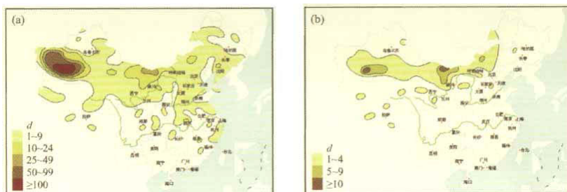
图2 2005年全国沙尘天气的空间分布：(a) 沙尘天气日数；(b) 沙尘暴日数
