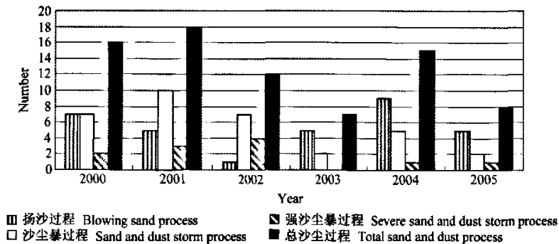
图3 2000~2005年春季全国各类沙尘天气过程次数及总次数
