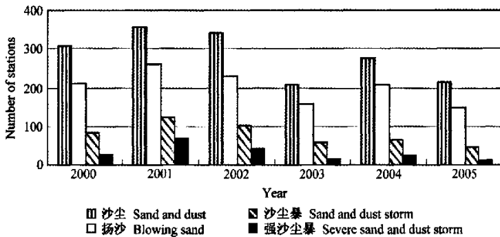
图 5 2000~2005 年春季全国沙尘天气总站数
