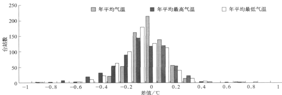
图 1 年平均、年平均最高、年平均最低气温差值频率分布图
