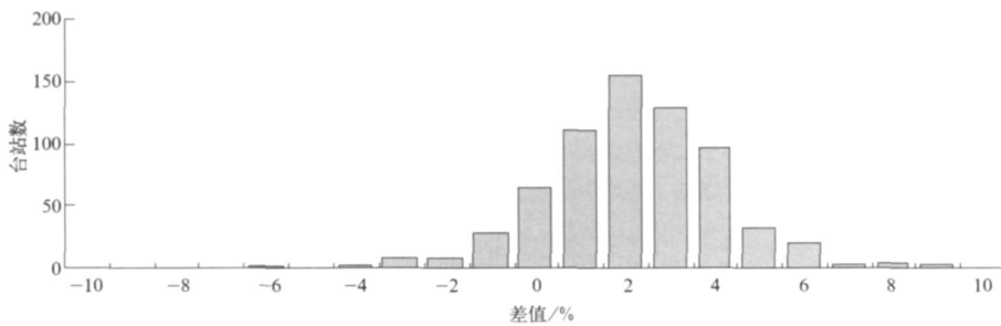
图2 相对湿度差值频率分布图
