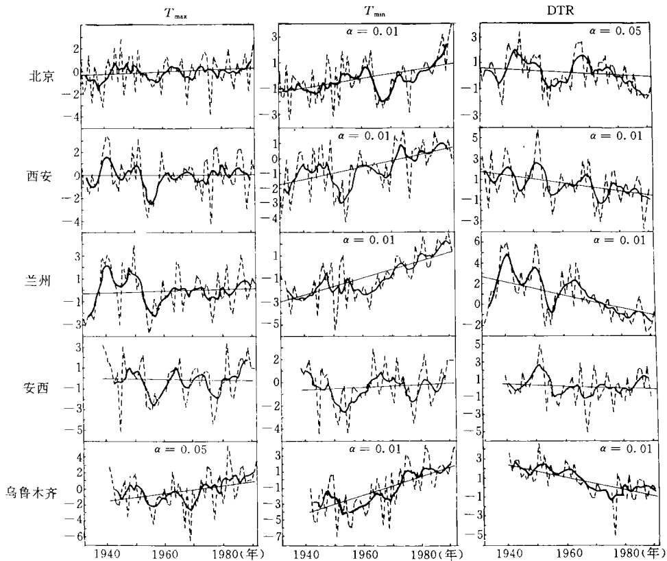
图 1 冬季西北地区及北京 T_{max} , T_{min} 及 DIR 变化曲线
