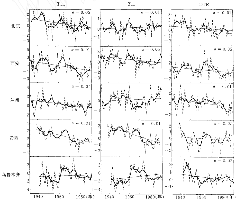
图 2 夏季西北地区及北京的 T_{\max} , T_{\min} , DTR 变化曲线
