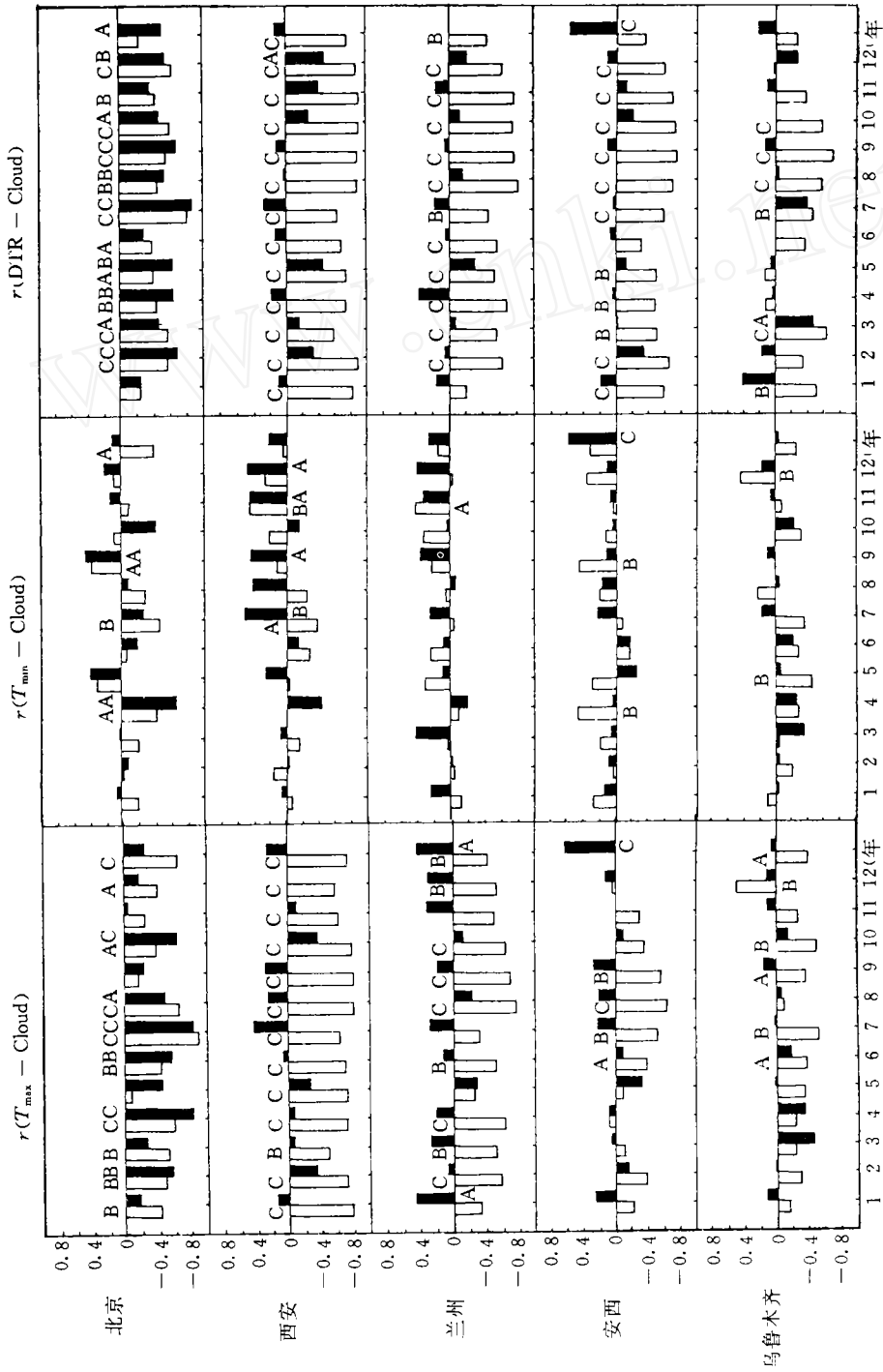
图3 1~12月及全年 T_{max} , T_{min} 及 DIR 与总云量和低云量的相关系数 (横坐标 1, 2, ..., 12 的单位为月, □ 为与总云量的相关分数, ■ 为与代云量的相关分数; A, \alpha=0.1 ; B, \alpha=0.05 ; C, \alpha=0.01 )
