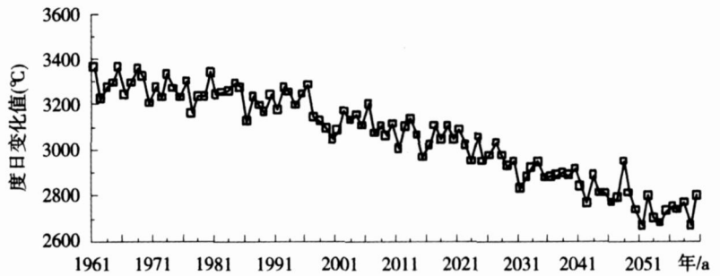
图 2 模式平均的我国年总度日
