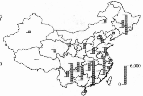
图 6 我国 2050~2059 年气候耗能的变化 (万吨标准煤)
