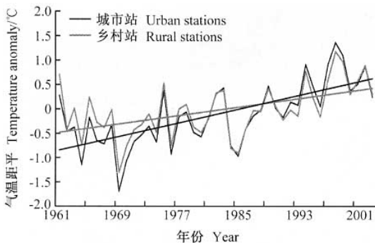
图 3 1961~2003 年期间河北省地区城市站、乡村站平均的年平均气温距平 Fig. 3 Annual mean air temperature anomalies for urban stations (US), rural stations (RS) over Hebei Province (1961—2003)
