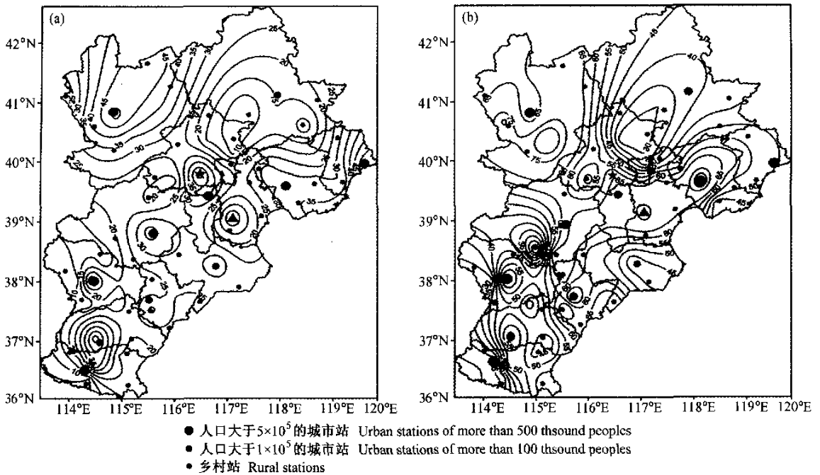
图5 河北省区域城市、乡村站年平均温度变化速率空间分布(单位: 10^{-2}/10\text{ a} )。(a) 1961~2003年; (b) 1981~2003年 Fig. 5 Spatial distribution of rates of annual mean air temperature change for urban stations (US), rural stations (RS) over Hebei Province (units; 10^{-2}/10\text{ a} ). (a) 1961—2003; (b) 1981—2003
