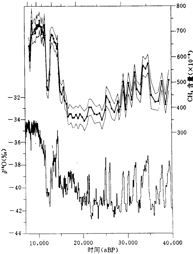
图 5 GRIP 冰芯记录在过去 4 万年氧同位素和大气 CH 4 含量 (引自 Chappellaz, et al, 1993) [11]
