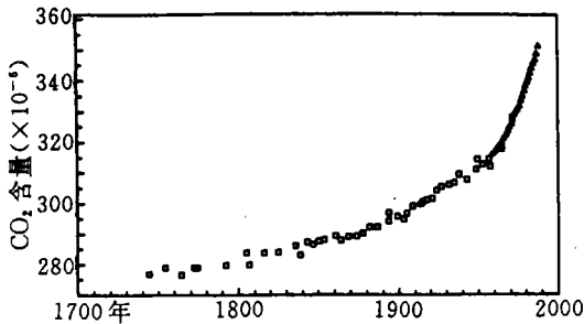
图 2 南极 Siple 站冰芯记录的过去 250 年大气 \text{CO}_2 含量变化与夏威夷 Mauna Loa 站仪器记录的大气 \text{CO}_2 含量变化 (引自 IPCC, 1990) [1]
