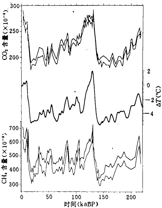
图 4 南极东方站冰芯记录的未来 22 万年大气 \text{CO}_2 、 \text{CH}_4 和温度变化 (Jouzel, et al, 1993) [8]
