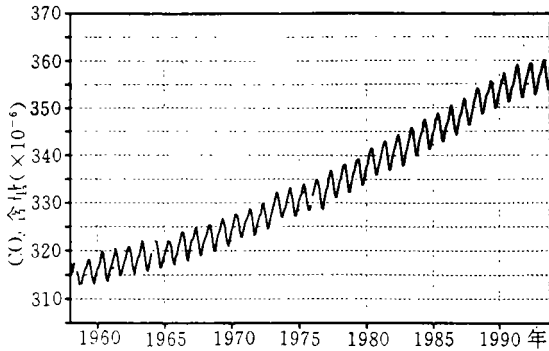
图 1 夏威夷 Mauna Loa 站的月平均大气 \text{CO}_2 含量记录 (1957~1993) (引自 WMO, 1994) [1~4]
