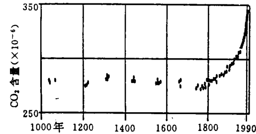
图 3 冰芯和直接测量得到的过去 1000 年大气 \text{CO}_2 含量变化 (引自 Lorius and Oeschger, 1994) [5]
